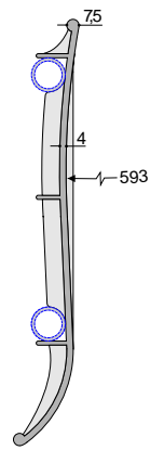
CORTE AA
