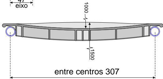
CORTE EE
