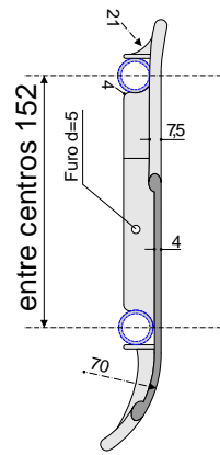
CORTE CC
