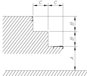
Figura 3 - Dimensões dos degraus.
