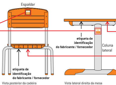
Vista posterior da cadeira
