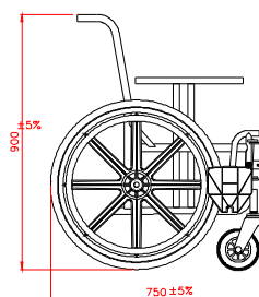
DETALHE CADEIRA PEDAL RECOLHIDO
